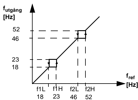
Figur 7 Exempel på inställning av kritiska frekvenser för ett fläktsystem som uppvisar kraftiga vibrationer i frekvensbanden 18 - 23 Hz och 46 - 52 Hz.
