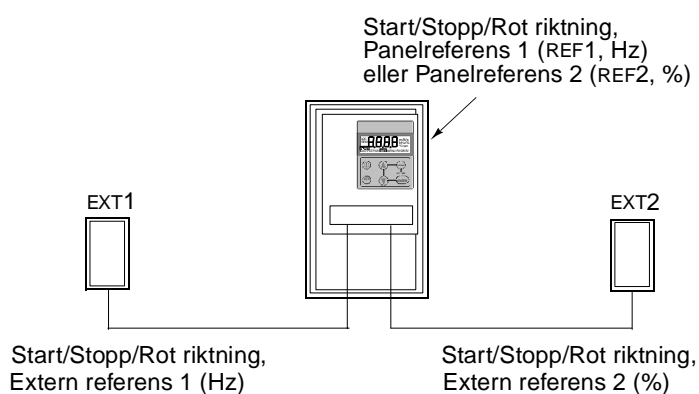
Figur 23 Styrplatser.
