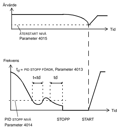
Figur 17 Vilofunktionens arbetssätt.
