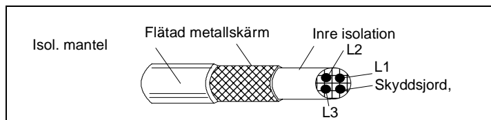
Figur 21 Effektiv motorkabelskärm (t ex Ölflex-Servo-FD 780 CP från Lappkabel eller MCCMK från NK Cables).
